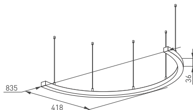
Рис. 1. Чертеж и габаритные размеры
