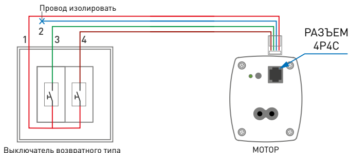
Рис. 2. Подключение мотора с помощью «сухих контактов»
