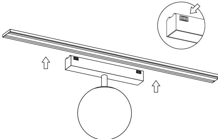
Рис. 2. Установка светильника
