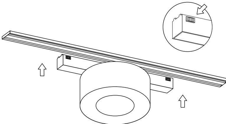
Рис. 2. Установка светильника
