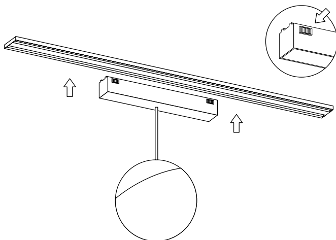
Рис. 2. Установка светильника
